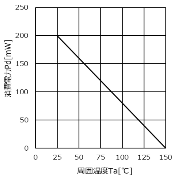
熱低減曲線
