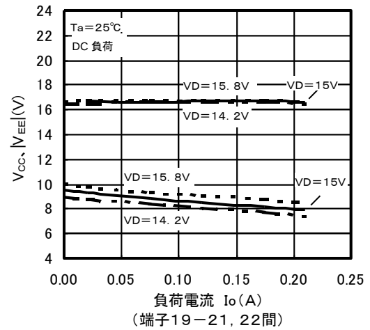
V_{CC} 、 |V_{EE}| - I_o 特性 (代表例)
