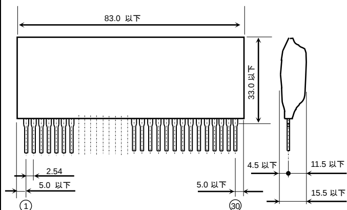
外形图
