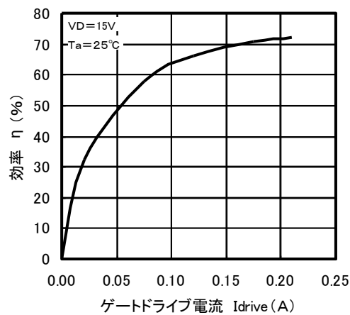
\eta - I_{drive} 特性 (代表例)
