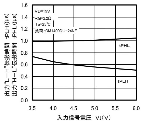
t_{PLH} 、 t_{PHL} - V_I 特性 (代表例)
