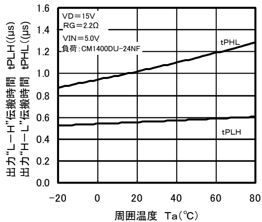
t_{PLH} 、 t_{PHL} - T_a 特性 (代表例)
