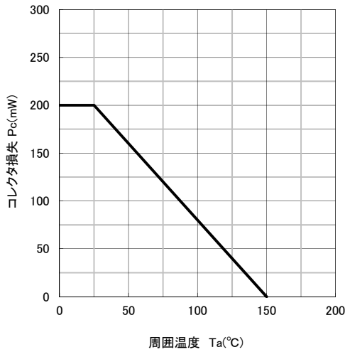
コレクタ損失-周囲温度特性
