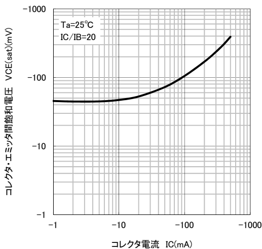
コレクタ・エミッタ間飽和電圧-コレクタ電流特性
