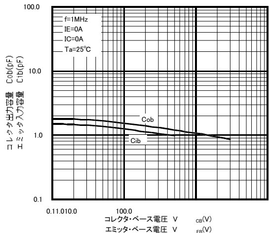
入出力容量—ベース電圧特性
