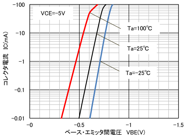
エミッタ接地伝達特性
