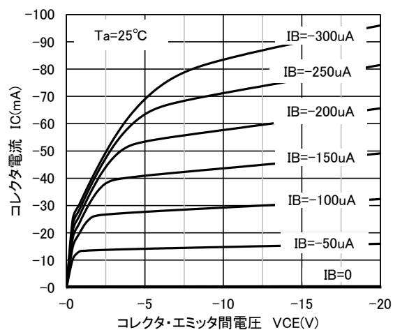
エミッタ接地出力特性
