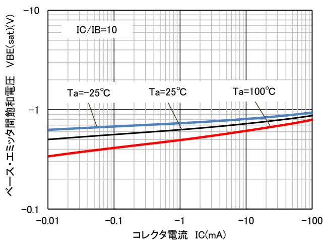
ベース・エミッタ間飽和電圧-コレクタ電流特性
