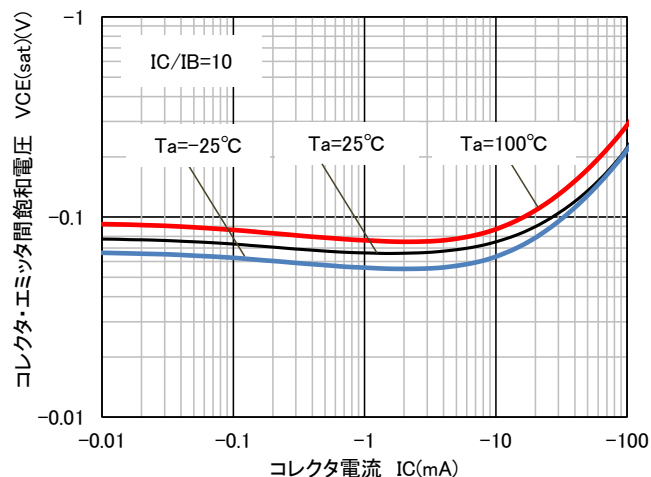
コレクタ・エミッタ間飽和電圧-コレクタ電流特性
