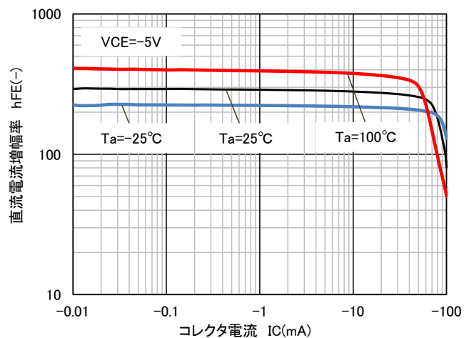
直流電流増幅率-コレクタ電流特性
