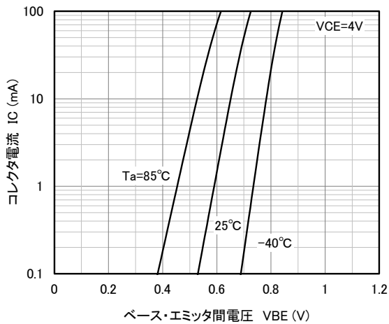
エミッタ接地伝達特性
