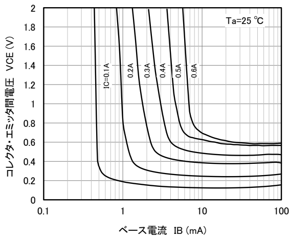
コレクタ・エミッタ間電圧-ベース電流特性
