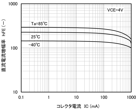
直流電流増幅率-コレクタ電流特性
