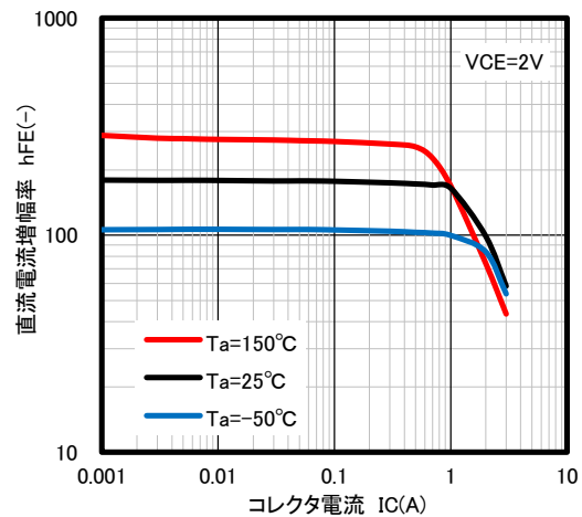
直流電流増幅率-コレクタ電流特性
