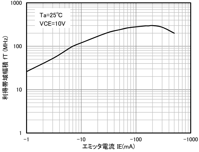
利得帯域幅積-エミッタ電流特性
