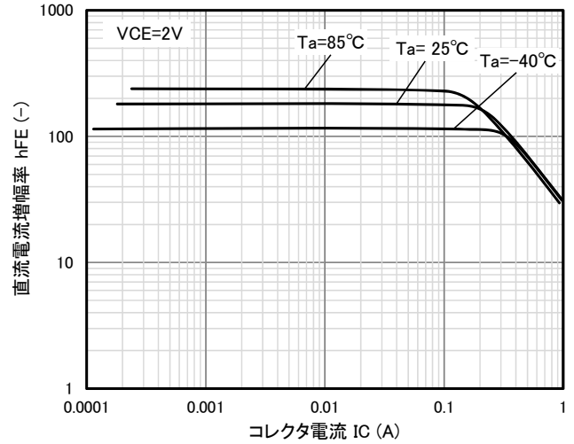
直流電流増幅率-コレクタ電流特性
