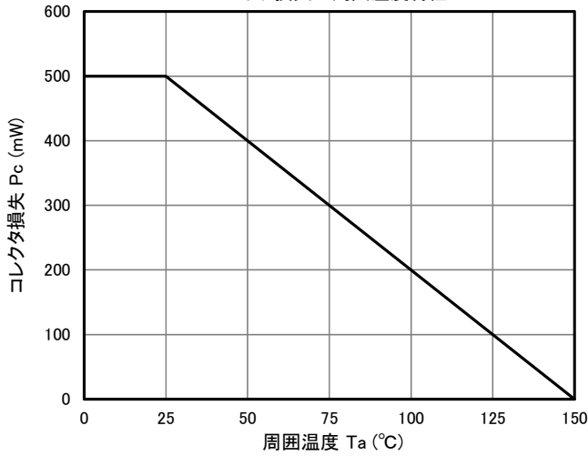
コレクタ損失-周囲温度特性
