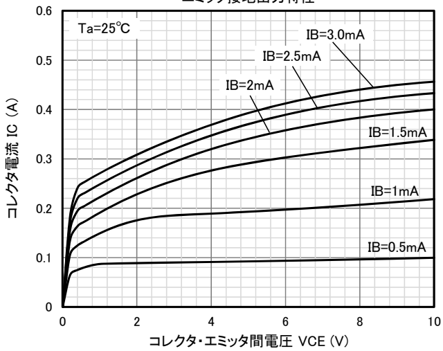
エミッタ接地出力特性
