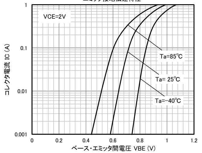
エミッタ接地伝達特性
