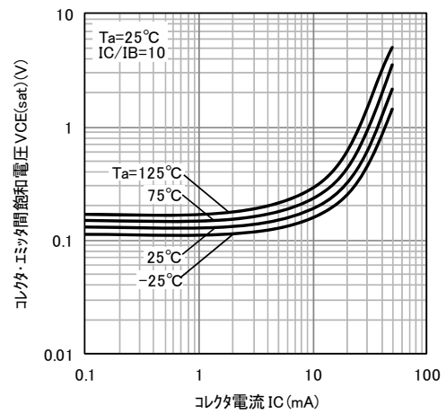
V_{CE(sat)}-I_C
