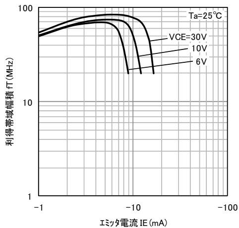
f_T-I_E
