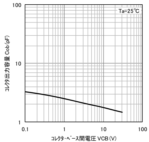
C_{ob}-V_{CB}
