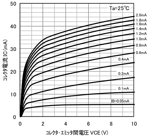
ミッタ接地出力特性
