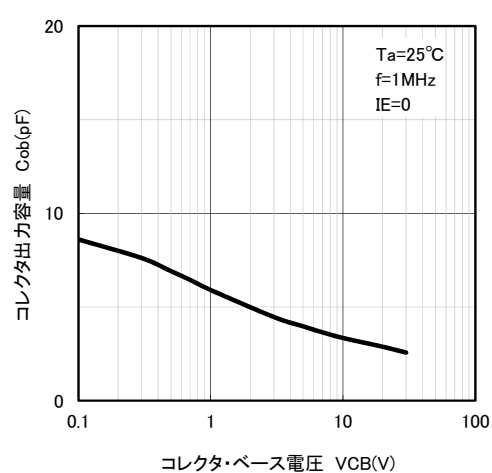
Cob-VCB特性グラフ
