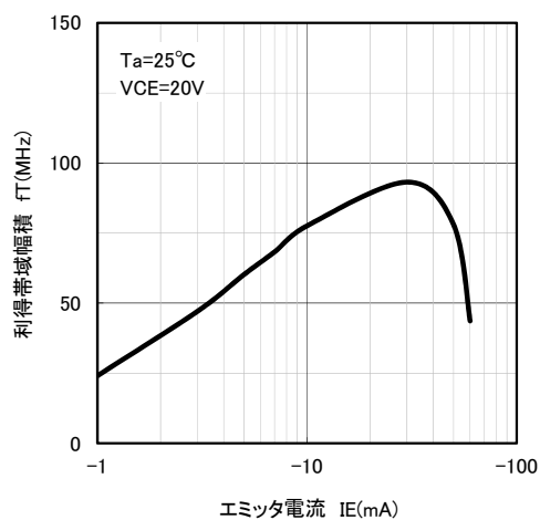
fT-IE特性グラフ
