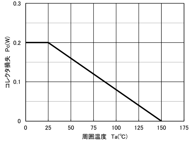
コレクタ損失-周囲温度特性
