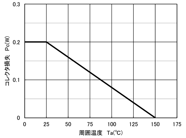
コレクタ損失-周囲温度特性
