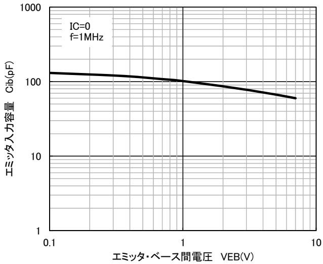
エミッタ入力容量-エミッタ・ベース間電圧特性
