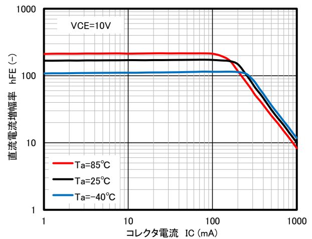
直流電流増幅率-コレクタ電流特性
