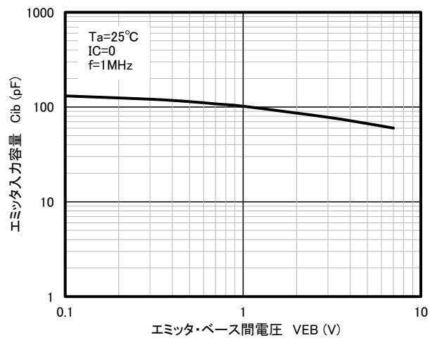
エミッタ入力容量-エミッタ・ベース間電圧特性
