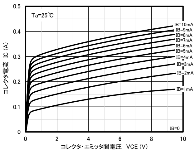
エミッタ接地出力特性
