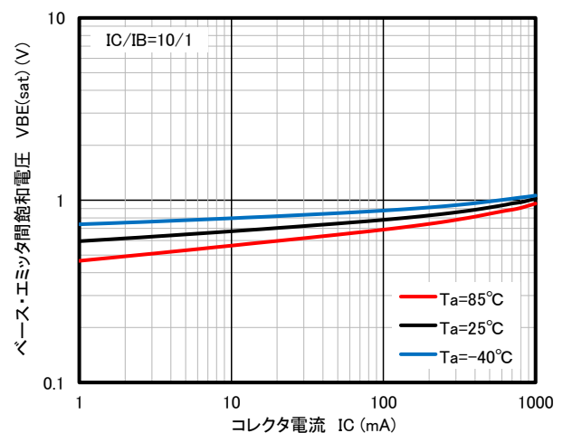
ベース・エミッタ間飽和電圧-コレクタ電流特性
