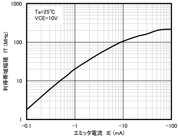
利得帯域幅積-エミッタ電流特性
