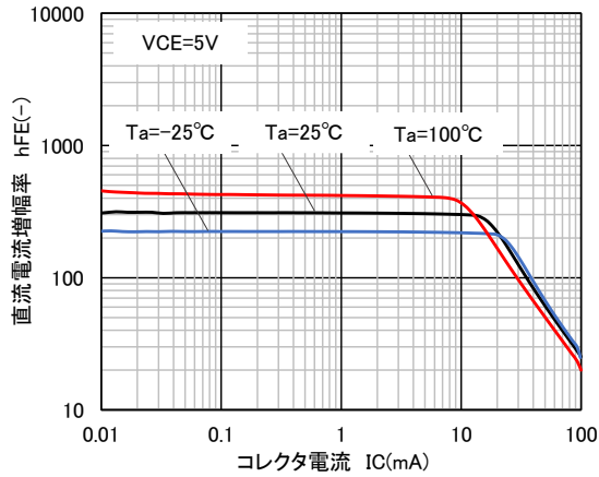
直流電流増幅率-コレクタ電流特性
