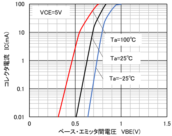
エミッタ接地伝達特性
