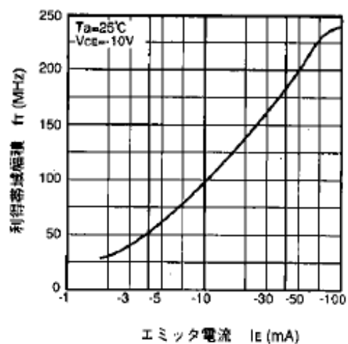
利得帯域幅積—エミッタ電流特性
