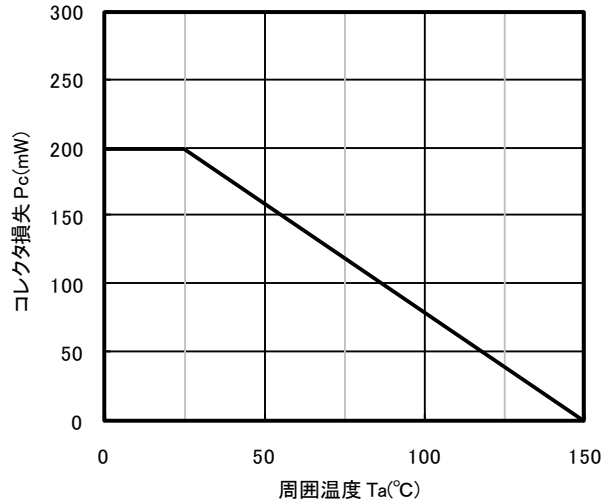
コレクタ損失－周囲温度特性
