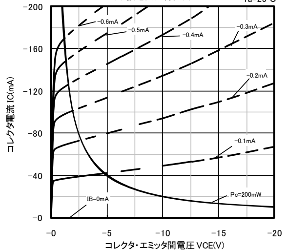
エミッタ接地出力特性(2) Ta=25°C
