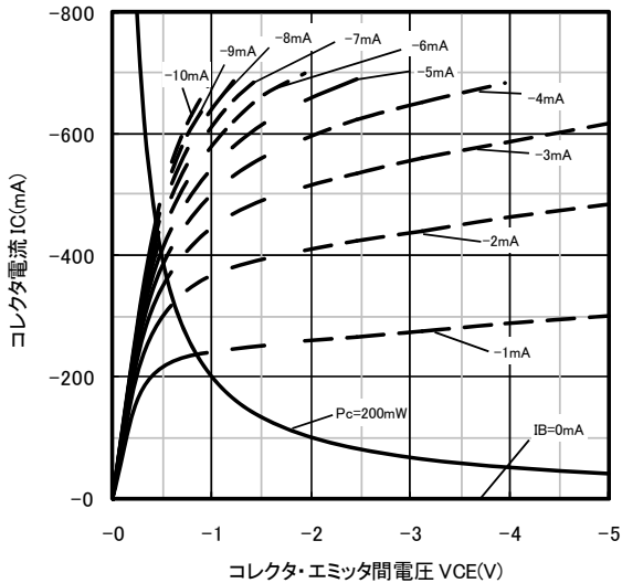
エミッタ接地出力特性(1) Ta=25°C
