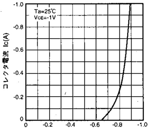
ベース・エミッタ間電圧 VBE(V)
