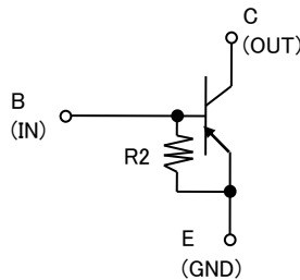
等価回路
