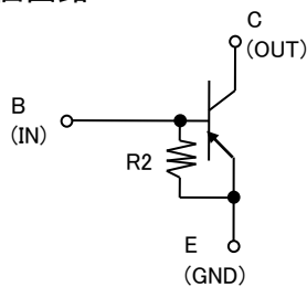
等価回路
