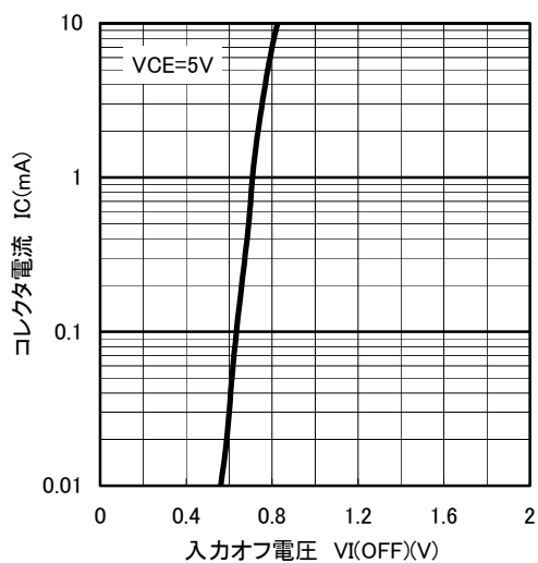
コレクタ電流－入力オフ電圧
