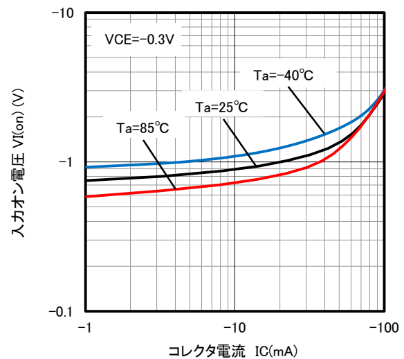
入力オン電圧-コレクタ電流
