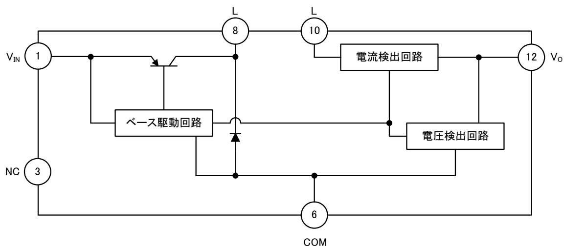
ブロック図
