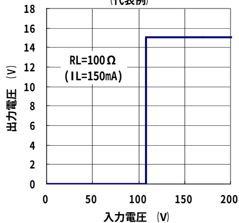
起動特性-1 (代表例)
