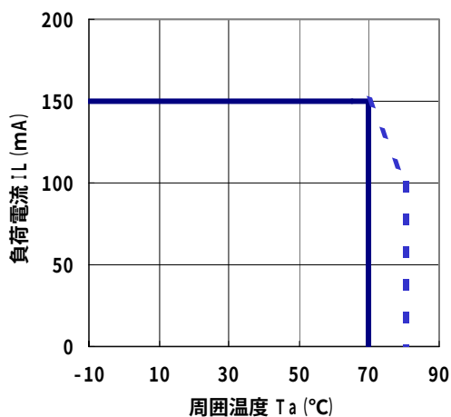
ディレーティング
