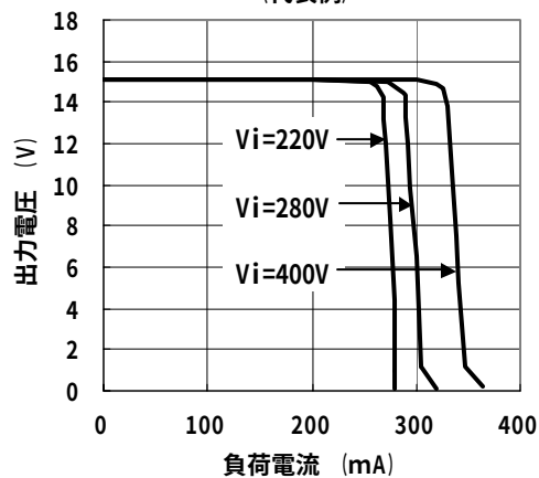
出力電圧-負荷電流特性 (代表例)
