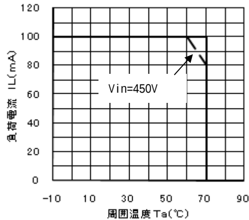
ディレーティング
