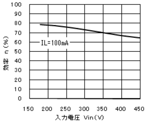
効率-入力電圧特性 （代表例）
