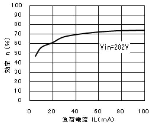
効率-負荷電流特性 （代表例）
