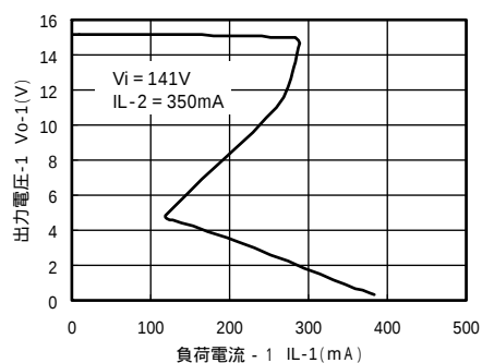
起動特性 - 1 (代表例)
