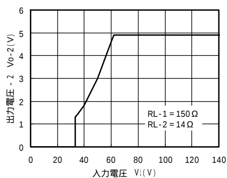
起動特性 - 2 (代表例)
