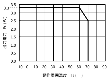
ディレーティング特性
