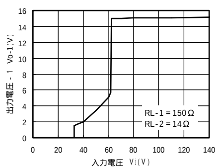
起動特性 - 1 (代表例)
