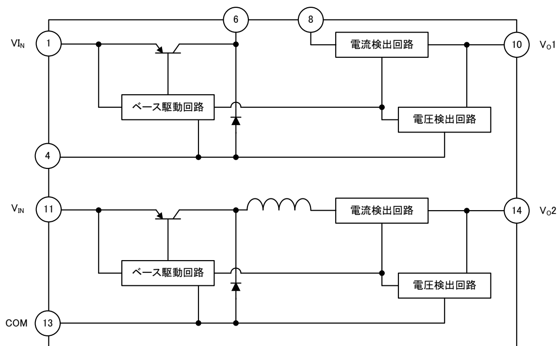
ブロック図
