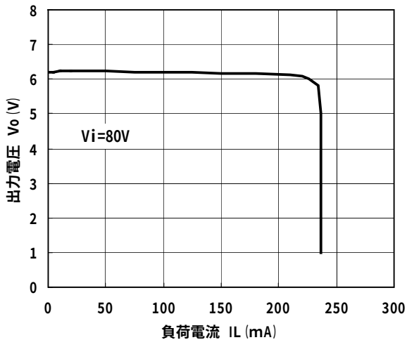
出力電圧-負荷電流特性 (代表例)
