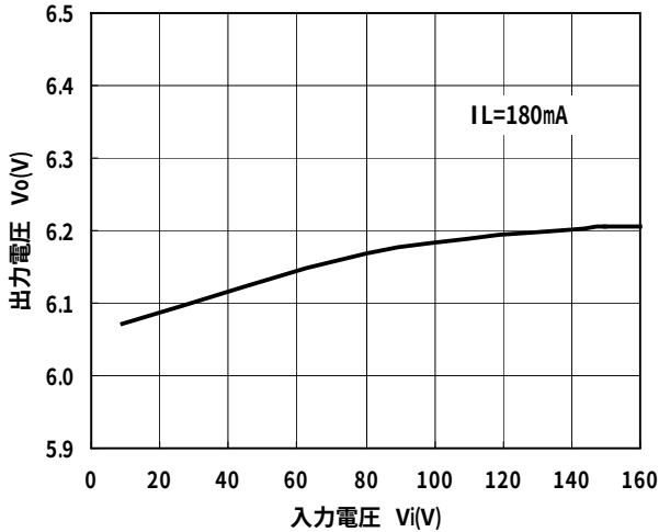
出力電圧-入力電圧特性 (代表例)
