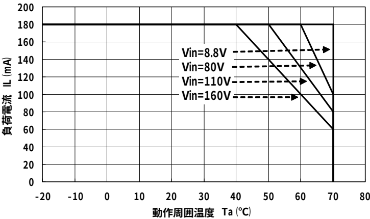
ディレーティング曲線
