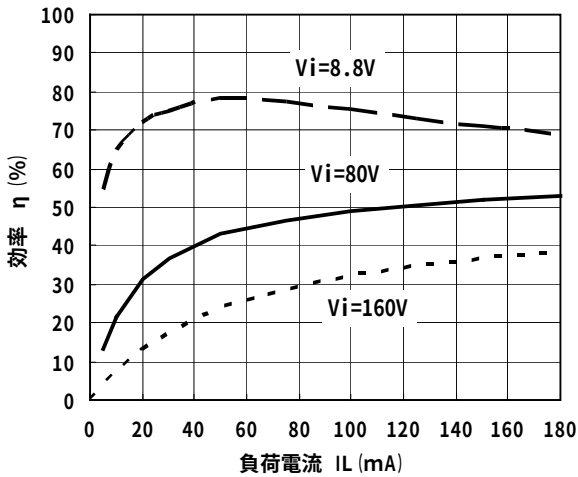
効率-負荷電流特性 (代表例)
