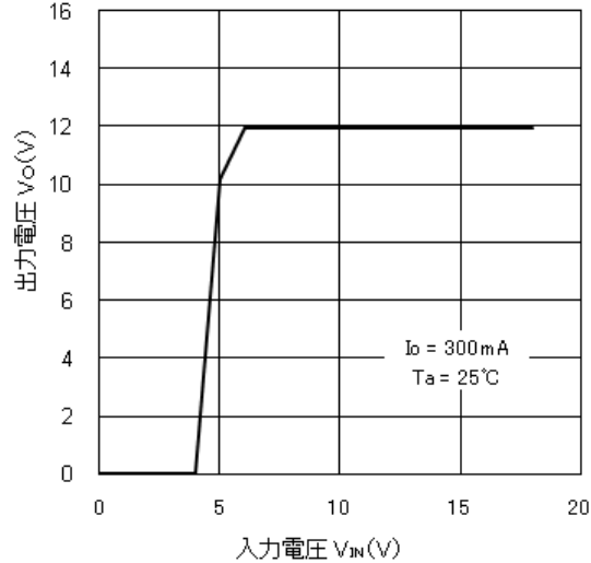
出力電圧 - 入力電圧特性
