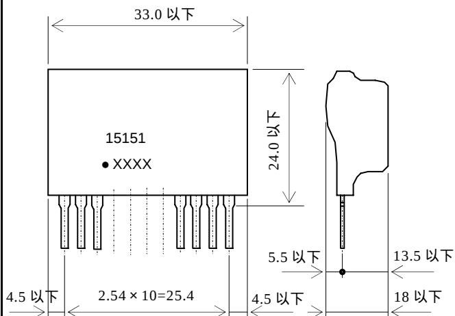
外形図
