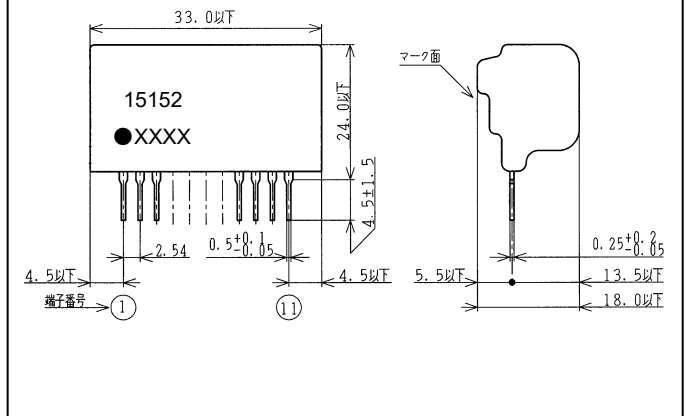
外形図
