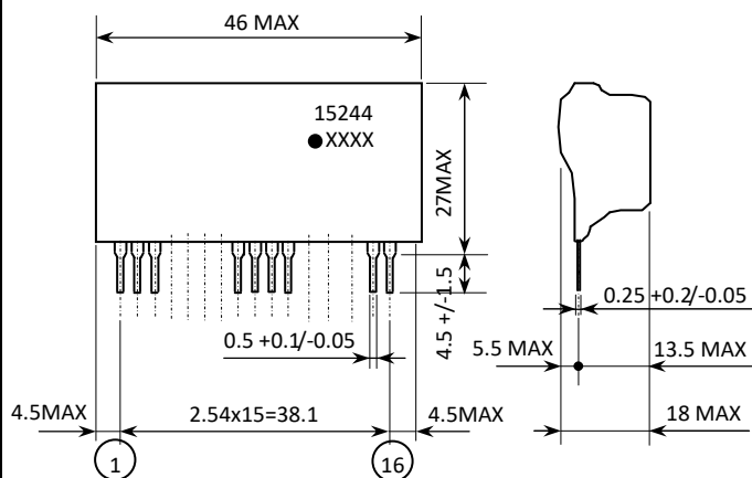
外形図
