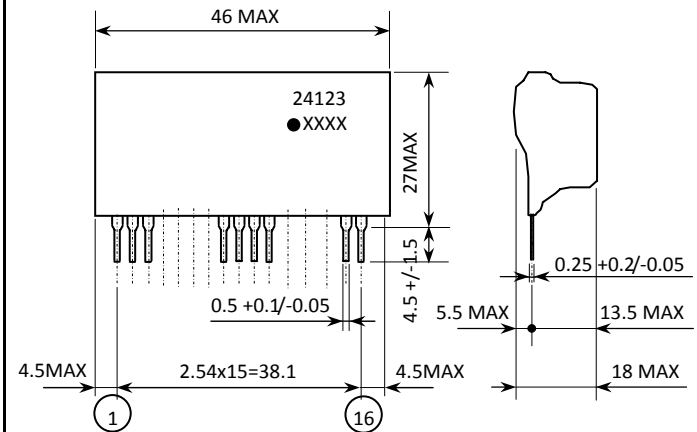
外形図
