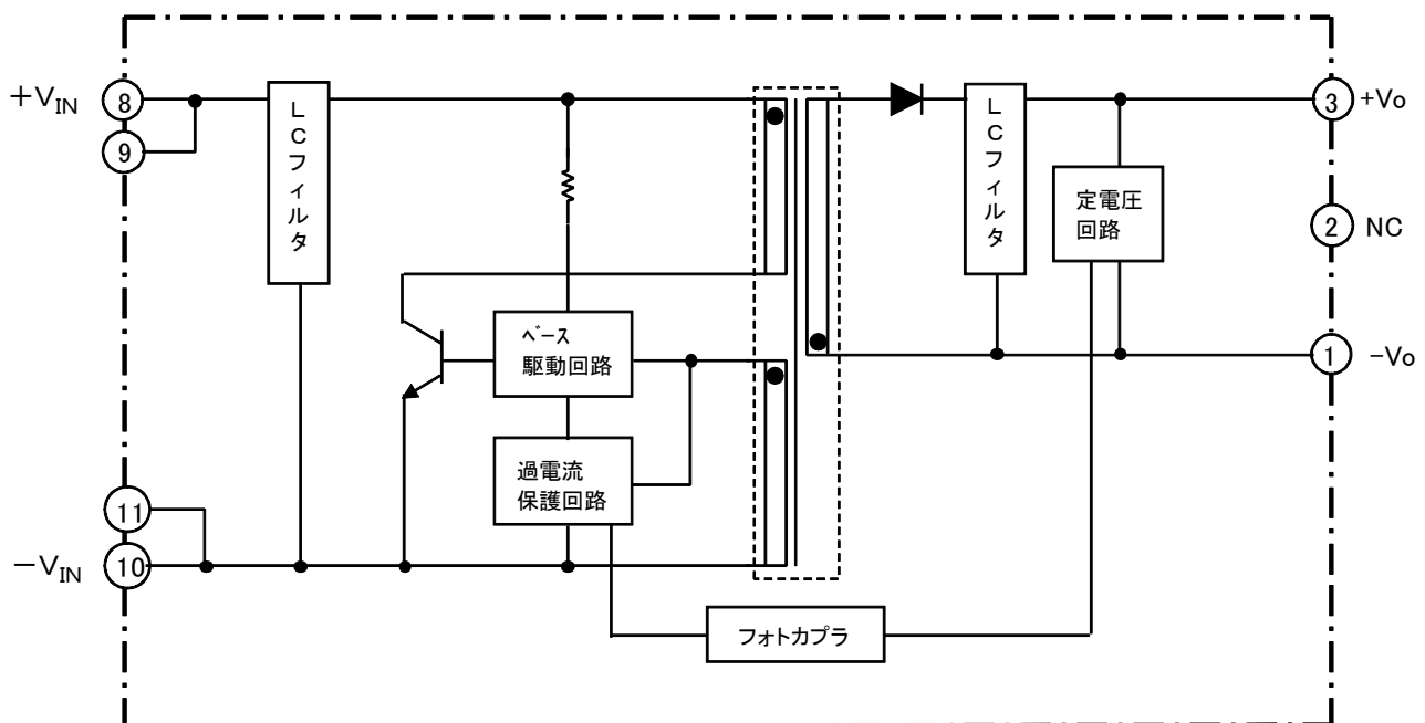
ブロック図
