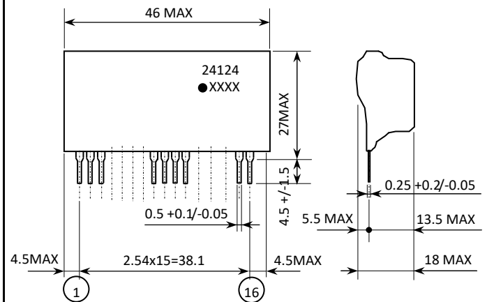
外形図
