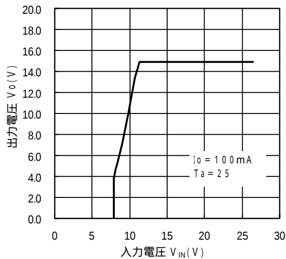
出力電圧 - 入力電圧特性
