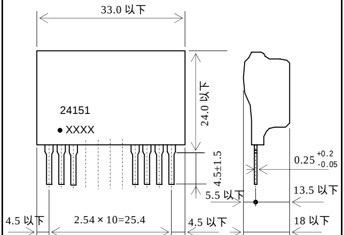
外形図
