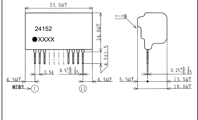
外形図
