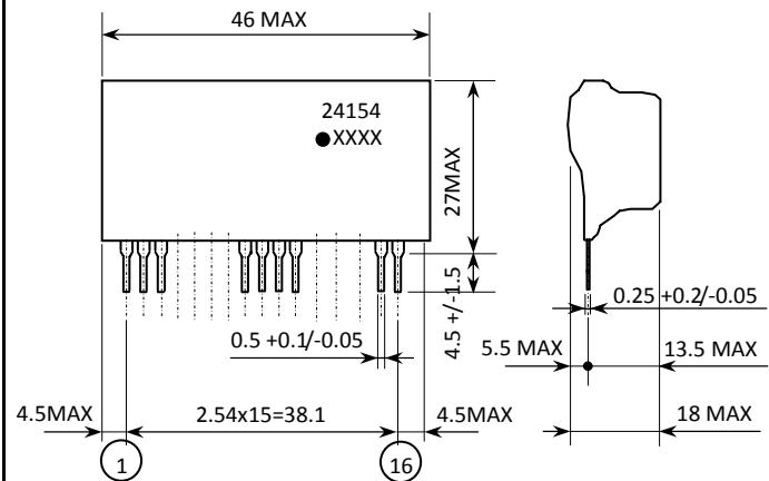
外形図
