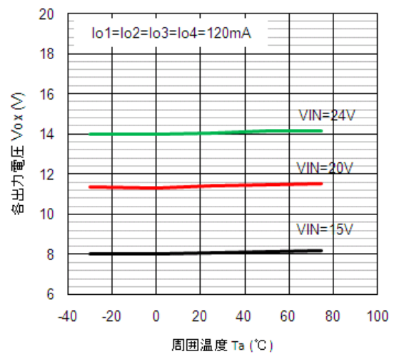
出力電圧 - 周囲温度特性
