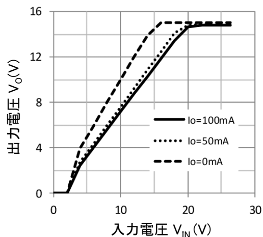
出力電圧—入力電圧特性1
