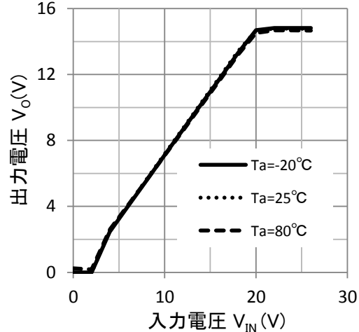
出力電圧—入力電圧特性2
