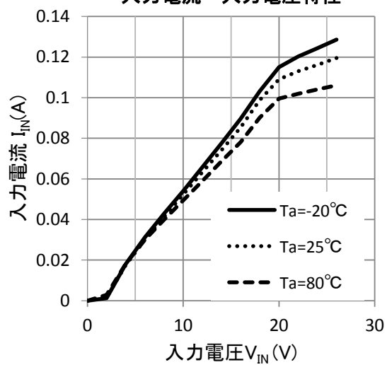
入力電流－入力電圧特性
