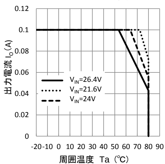
デレレーティング特性
