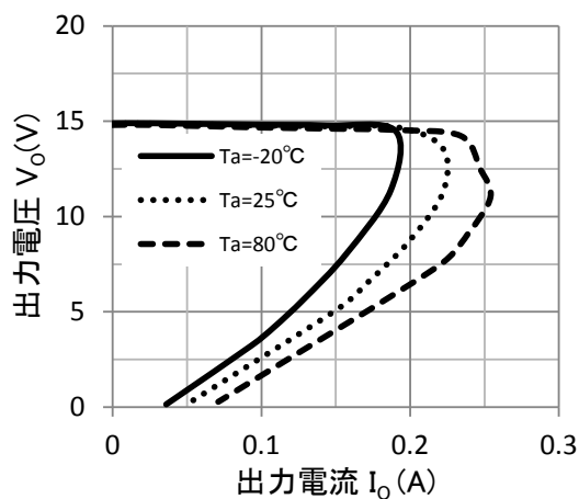
過電流保護特性
