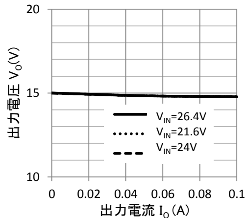
出力電圧—出力電流特性
