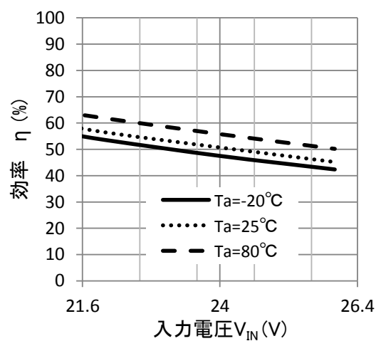
効率—入力電圧特性
