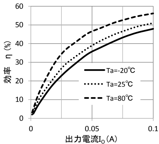
効率—出力電流特性
