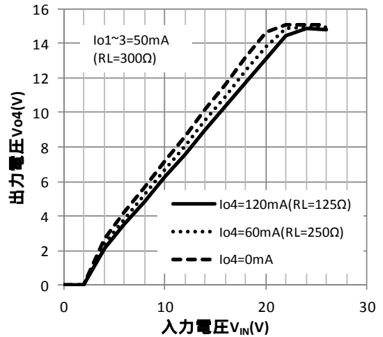
出力電圧4-入力電圧特性
