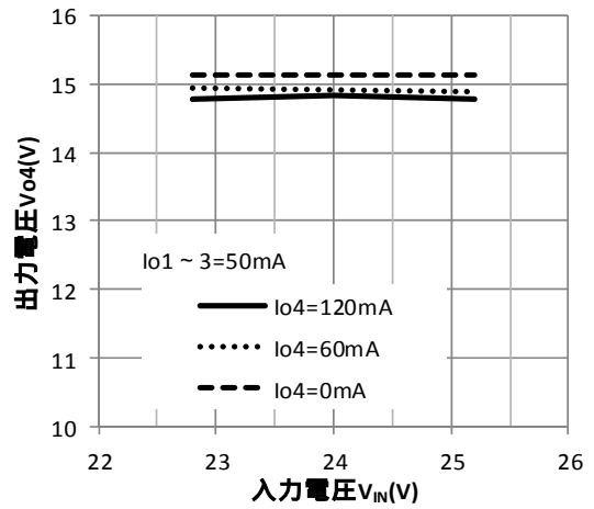
出力電圧4-入力電圧特性
