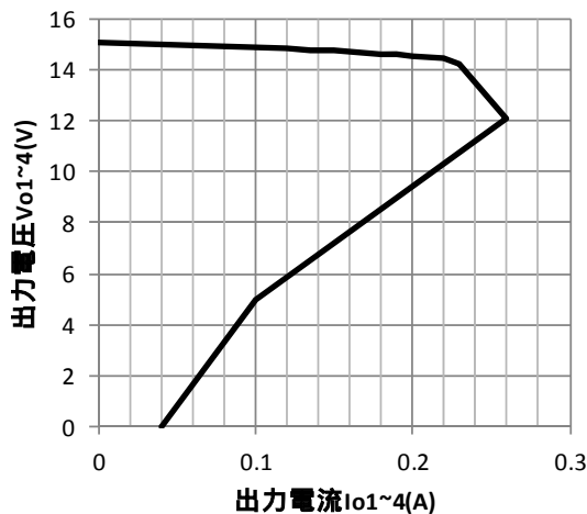
過電流保護特性
