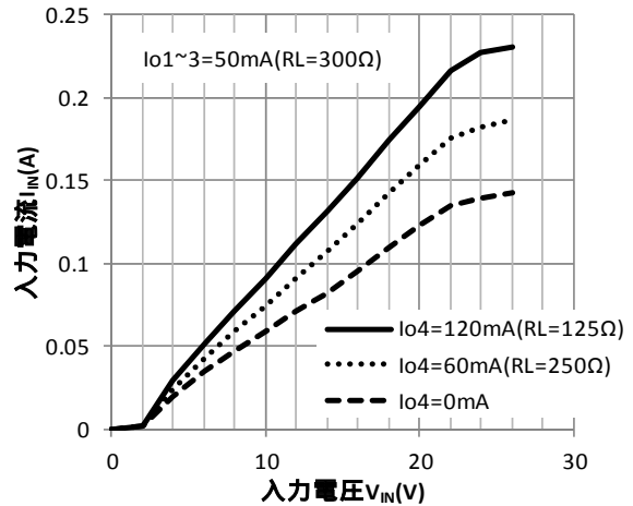
入力電流-入力電圧特性
