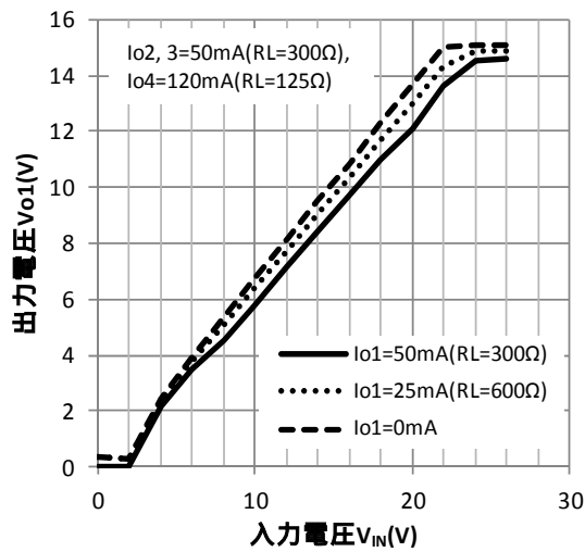
出力電圧1-入力電圧特性
