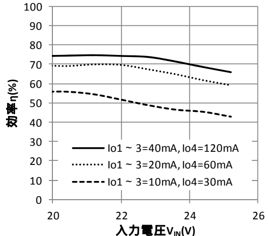
効率-入力電圧特性
