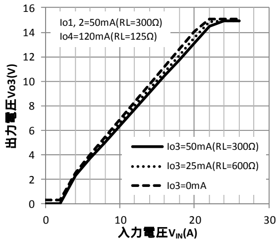
出力電圧3-入力電圧特性
