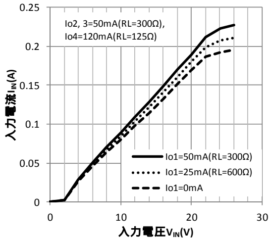
入力電流-入力電圧特性
