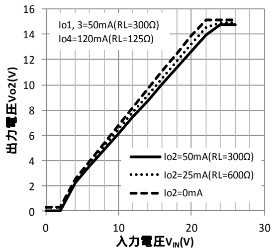
出力電圧2-入力電圧特性
