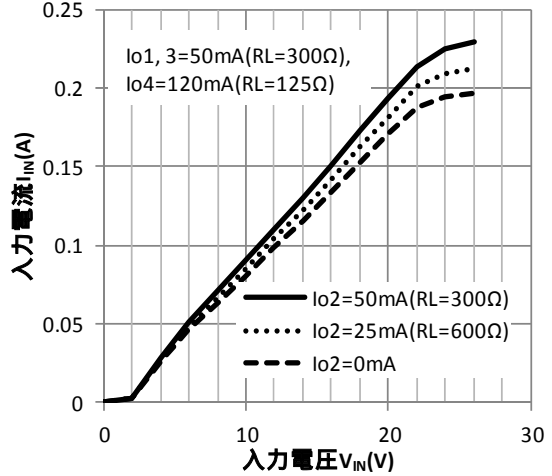
入力電流-入力電圧特性
