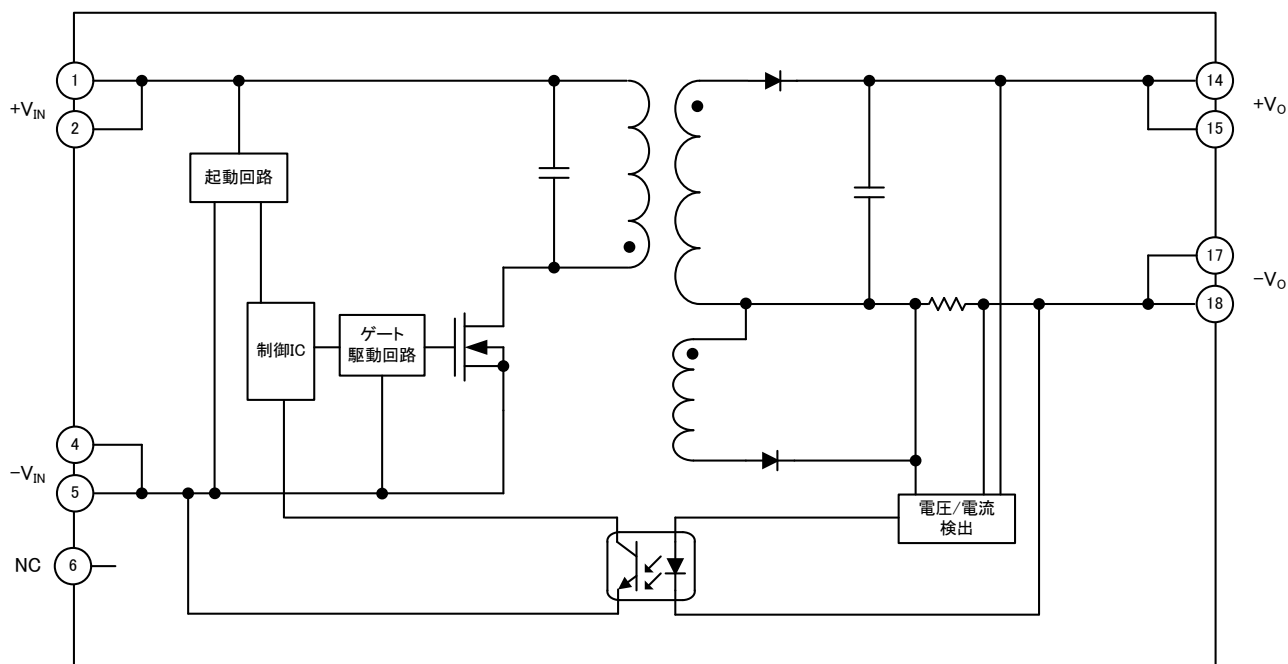
ブロック図
