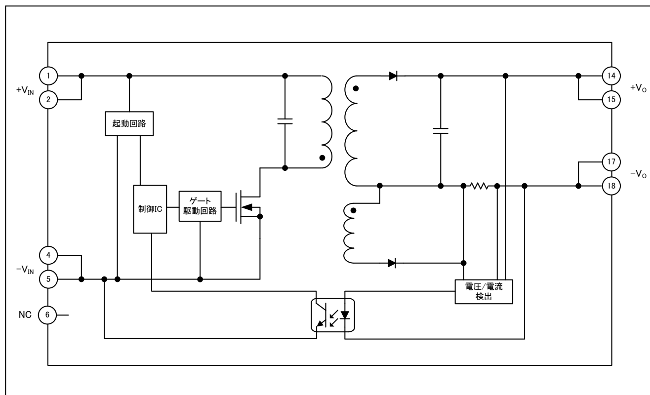
ブロック図
