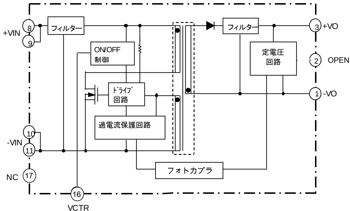
ブロック図
