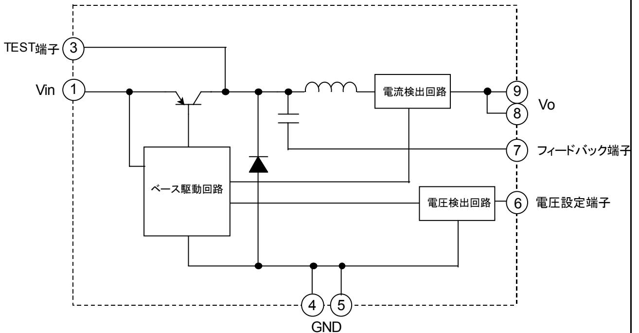
ブロック図
