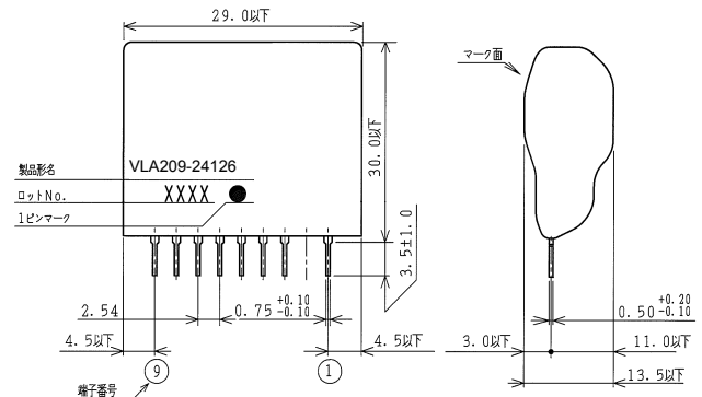
外形図
