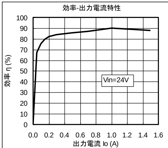
特性曲線【代表例】（出力電圧設定12V時）（ T_a=25^\circ\text{C} ）
