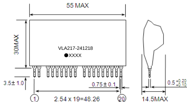
外形図
