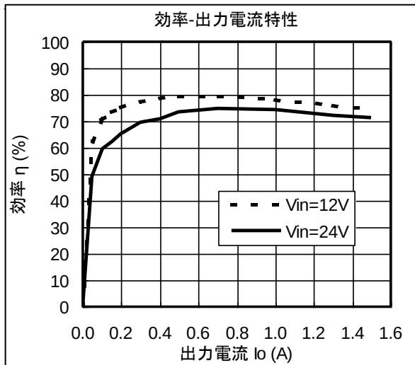
特性曲線【代表例】（出力電圧設定3.3V時）（ T_a=25^\circ\text{C} ）
