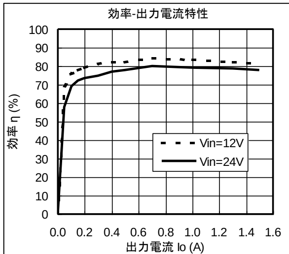
特性曲線【代表例】（出力電圧設定5V時）（ T_a=25^\circ\text{C} ）
