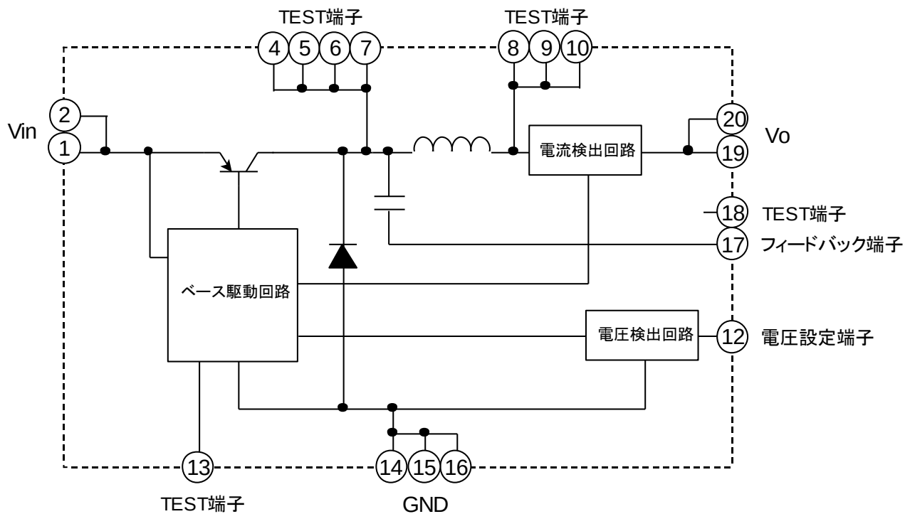
ブロック図
