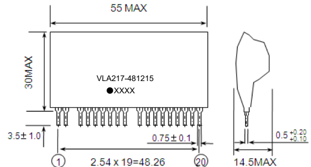
外形図
