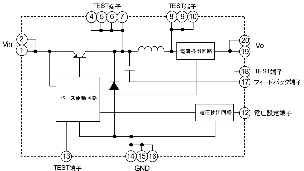
ブロック図
