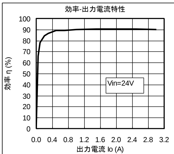
特性曲線【代表例】（出力電圧設定12V時）（ T_a=25^\circ\text{C} ）
