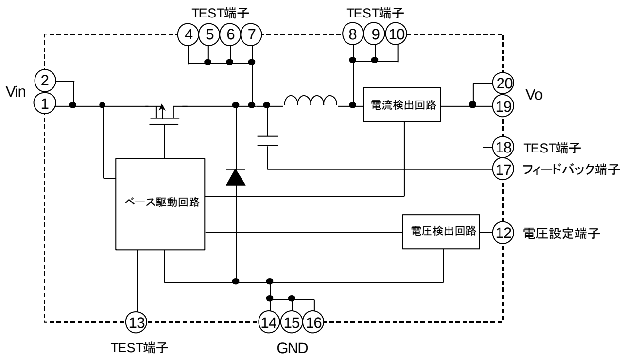
ブロック図
