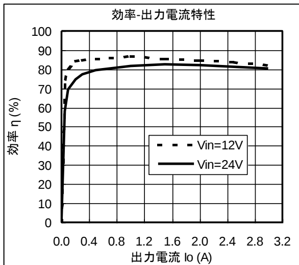
特性曲線【代表例】（出力電圧設定5V時）（ T_a=25^\circ\text{C} ）
