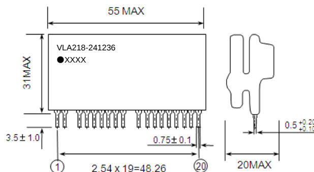
外形図
