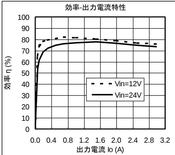
特性曲線【代表例】（出力電圧設定3.3V時）（ T_a=25^\circ\text{C} ）
