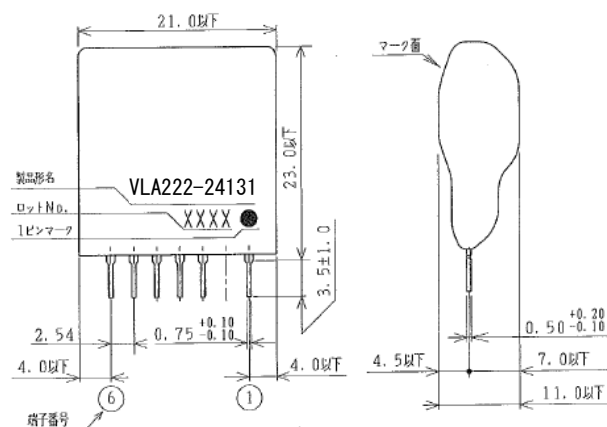
外形図
