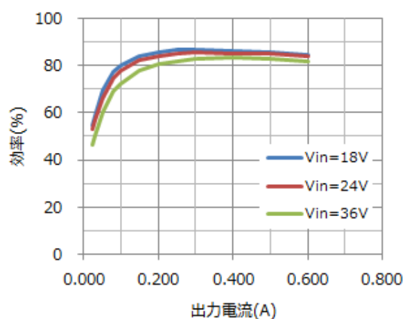
効率-出力電流特性
