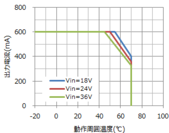
デレーティング特性
