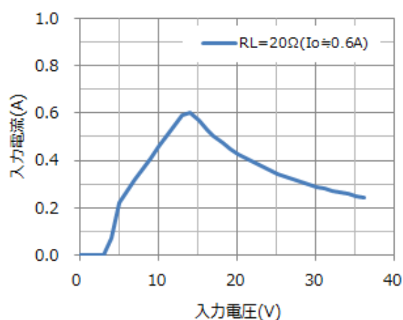
入力電流-入力電圧特性
