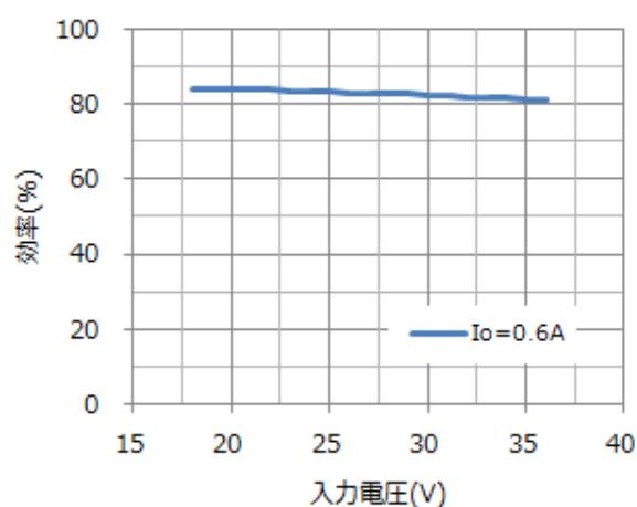
効率-入力電圧特性
