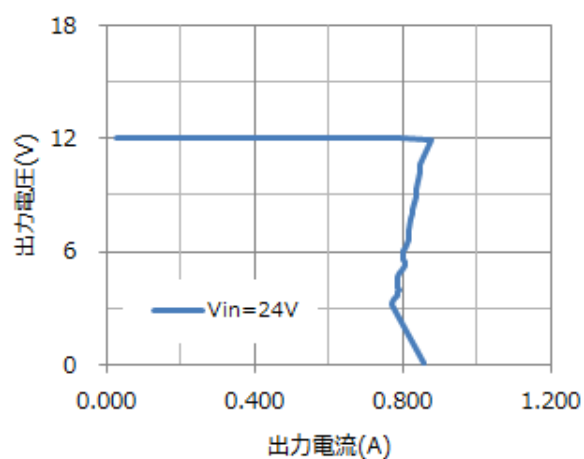
出力電圧-出力電流特性
