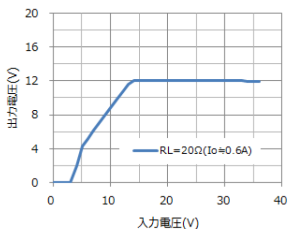
出力電圧-入力電圧特性
