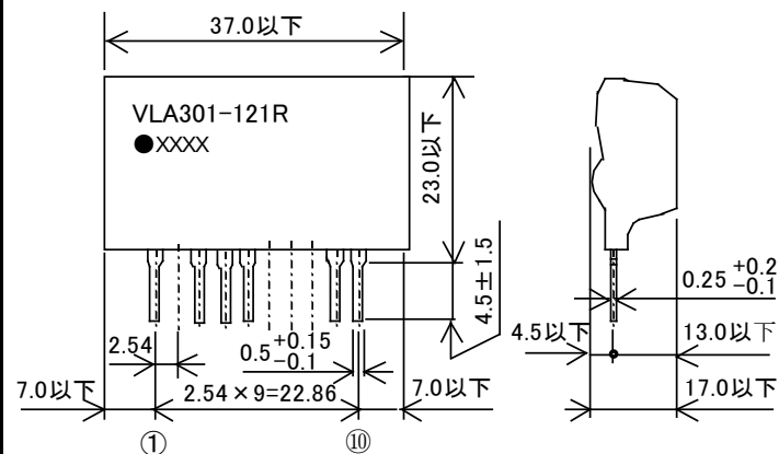
外形図
